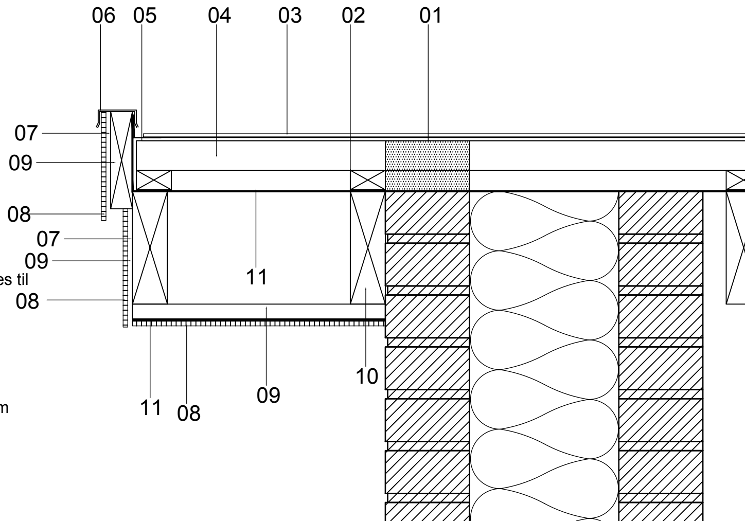
Lodret snit - Gavl
