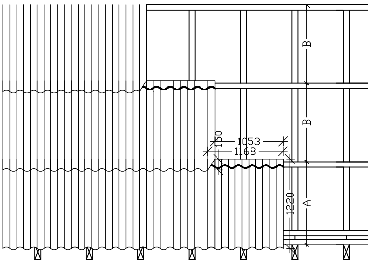
Tagplader oplagt 1:50
