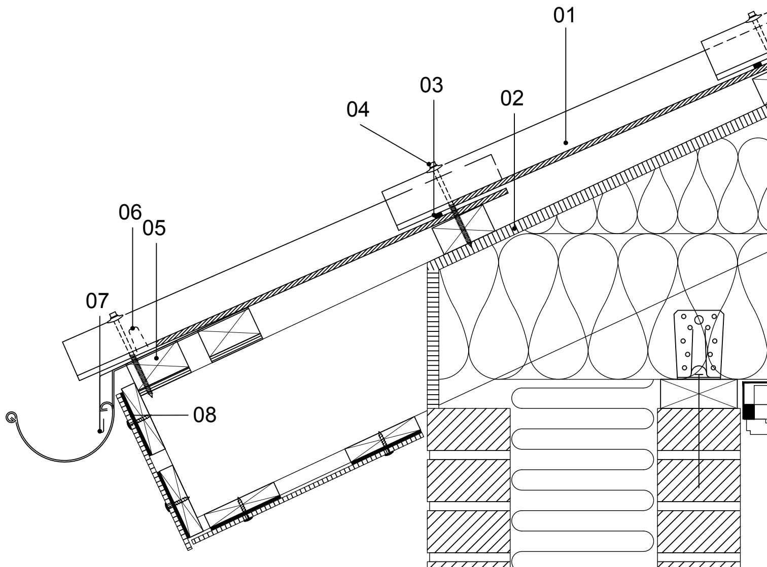
Lodret snit - tagfod uden undertag
